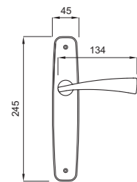
DO 10 maniglia su placca door handle on plate
