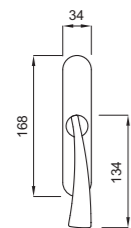
DO 20 cremonese con meccanismo window handle with mechanism
